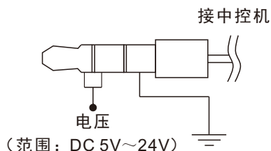
3.5mm耳机插头接线示意图
